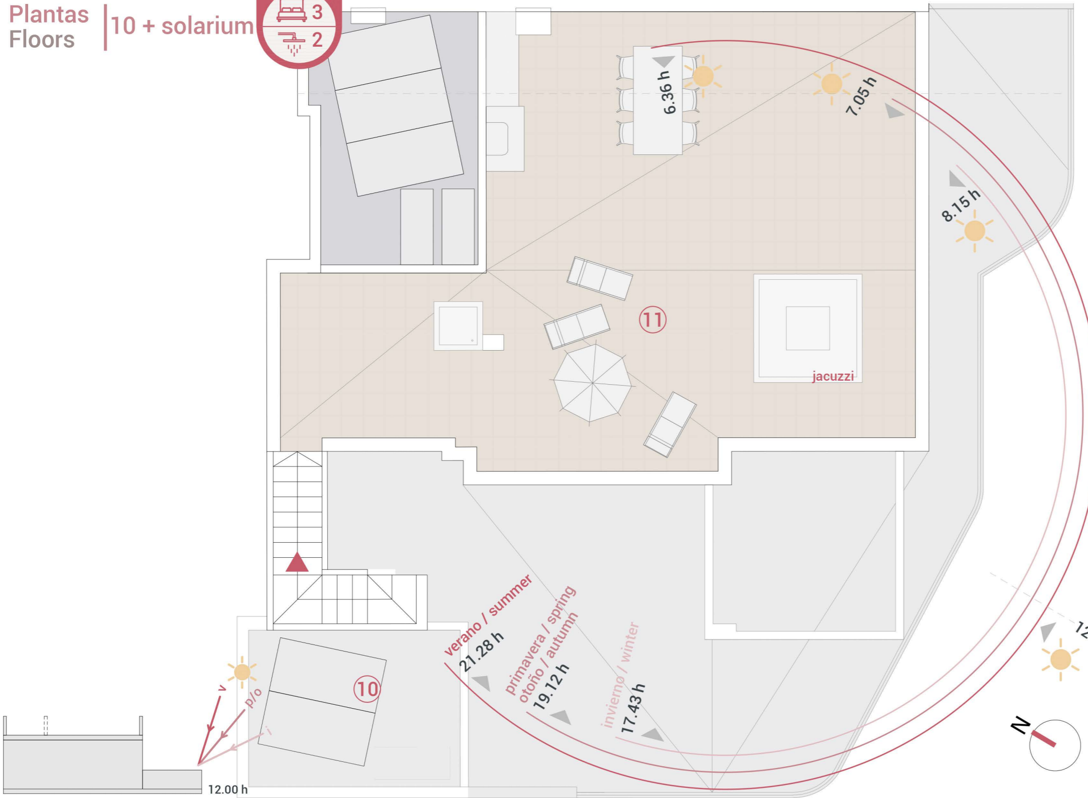
TIPO 0: 3D+2B PLANTA 10.ª TI
