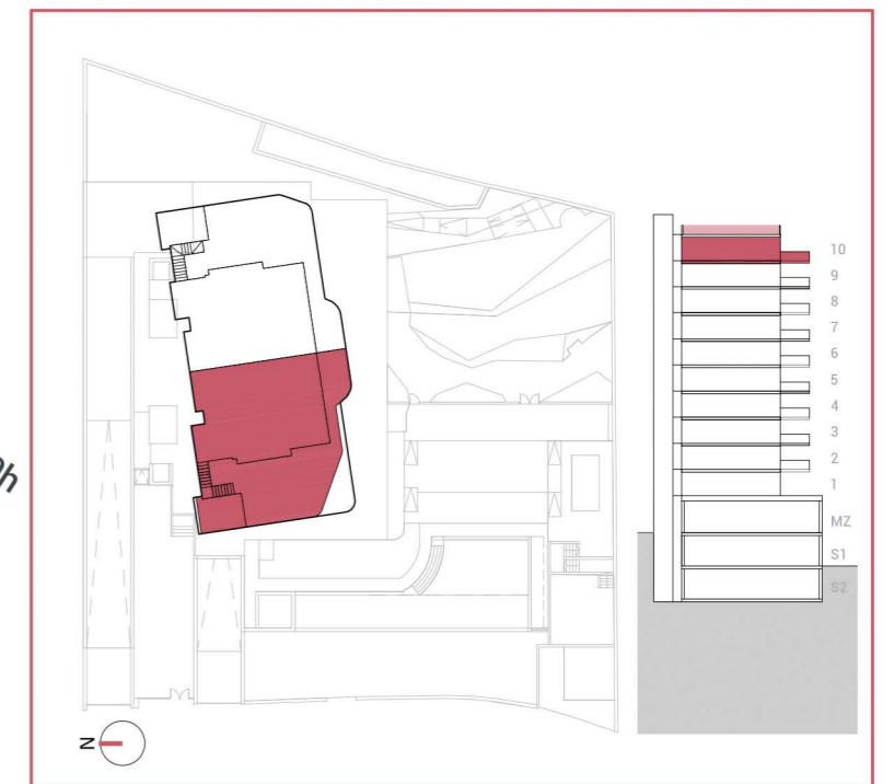
TIPO 0: 3D+2B PLANTA 10.ª TI
