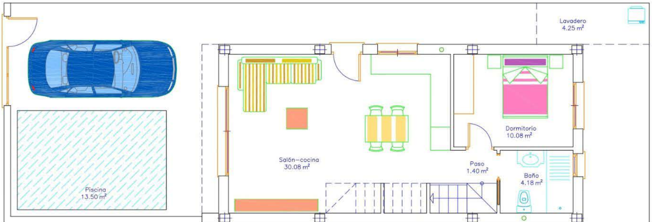
PLANTA BAJA S.C. VIVIENDA= 59.40M2 S.C. LAVADERO= 4.35M2
