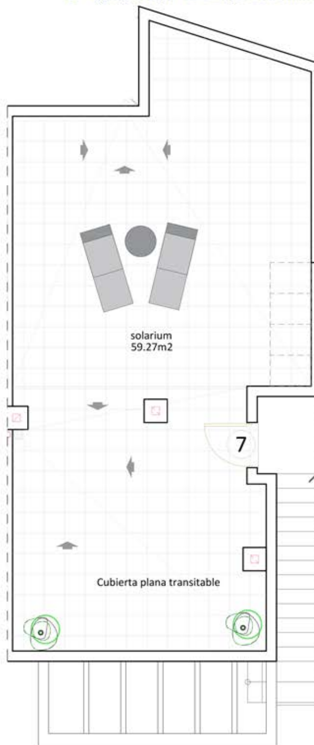
PLANTA SOLARIUM
