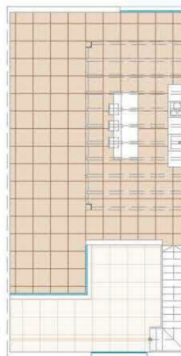
First Floor/ Planta Primera (E:1/100)
