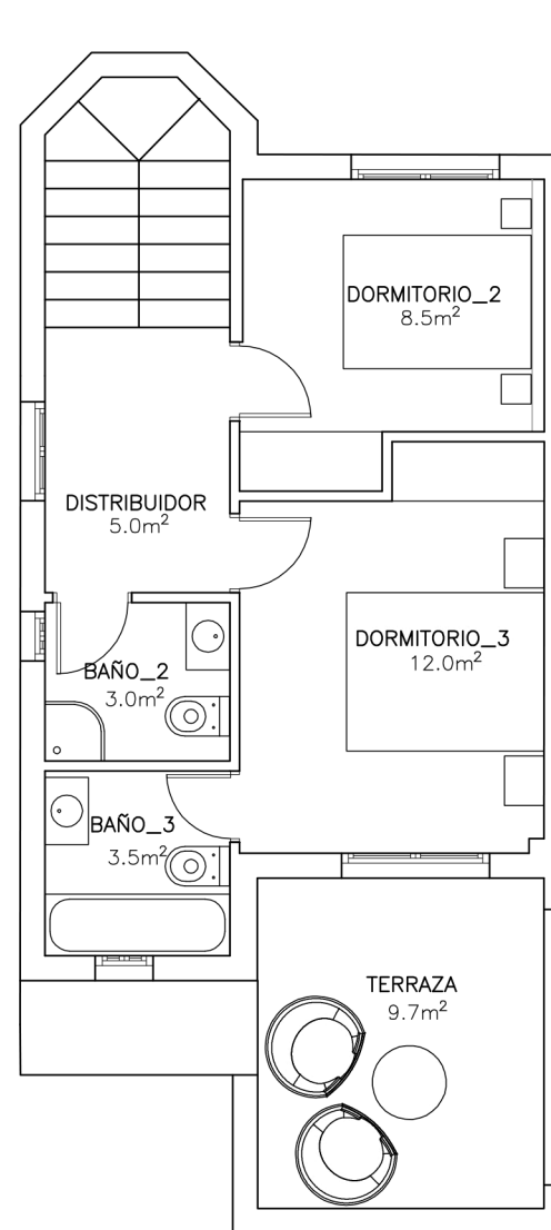
PLANTA PRIMERA
