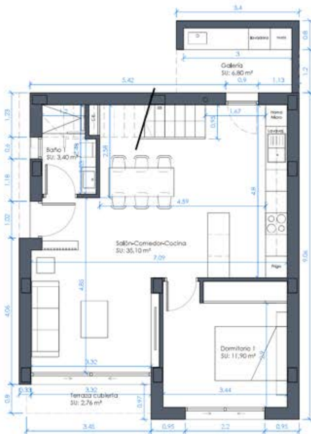
PLANTA BAJA
