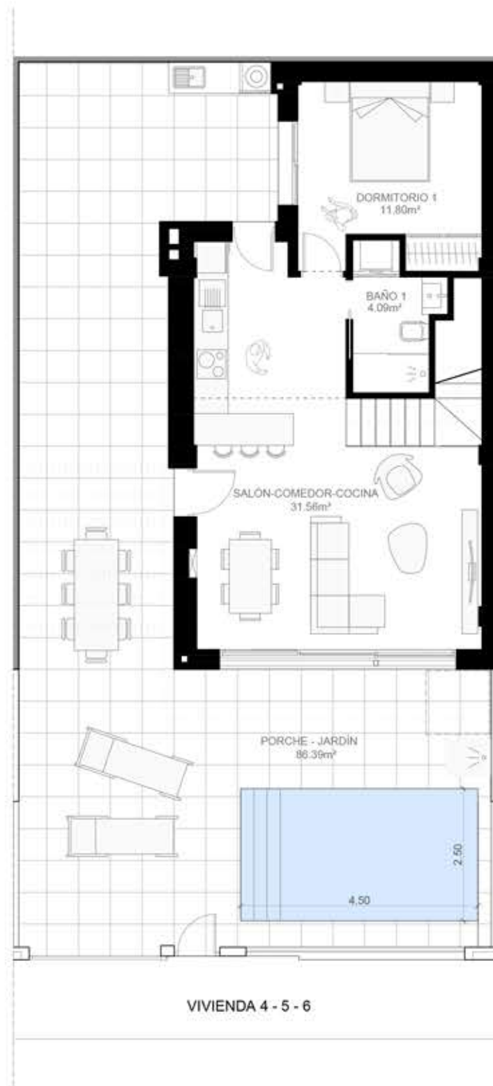
PLANTA BAJA
