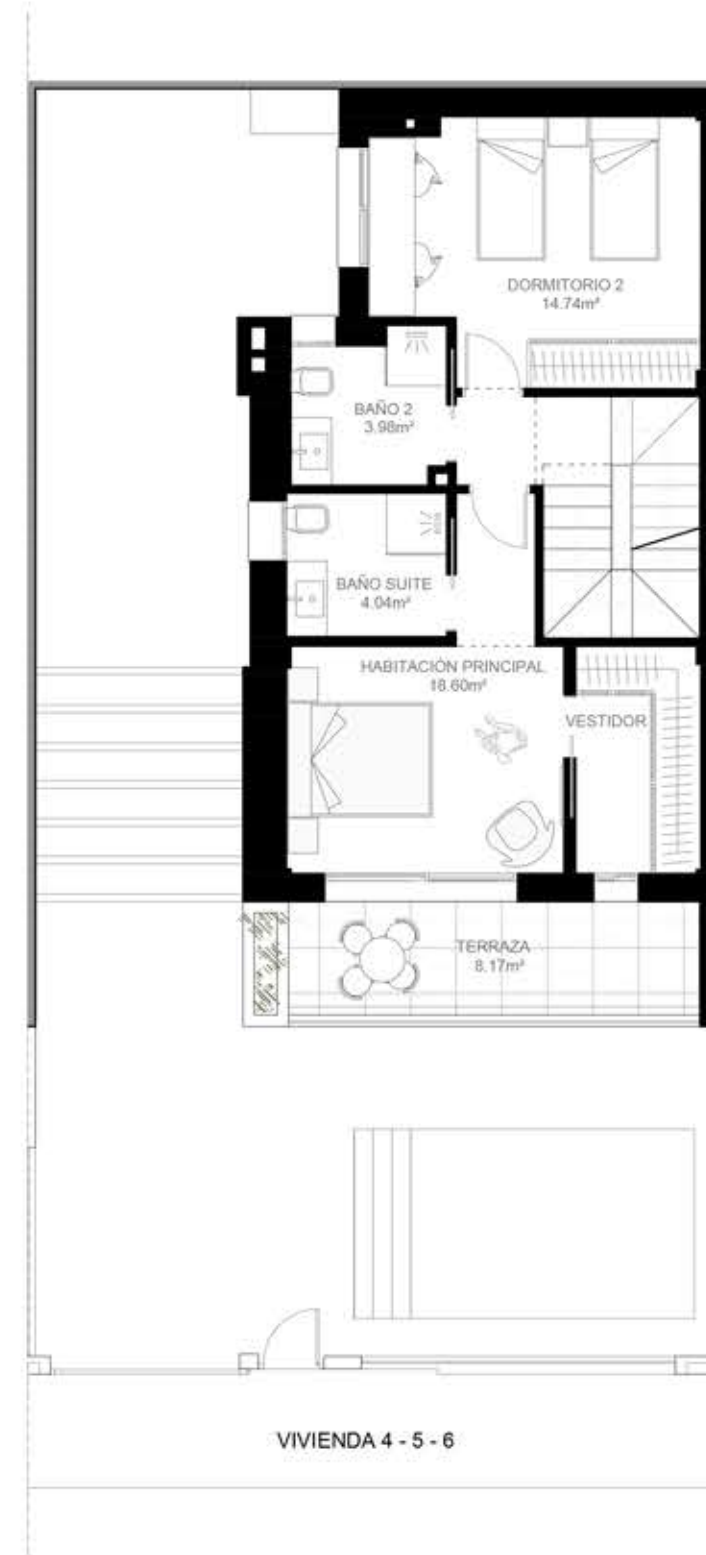
PLANTA PRIMERA
