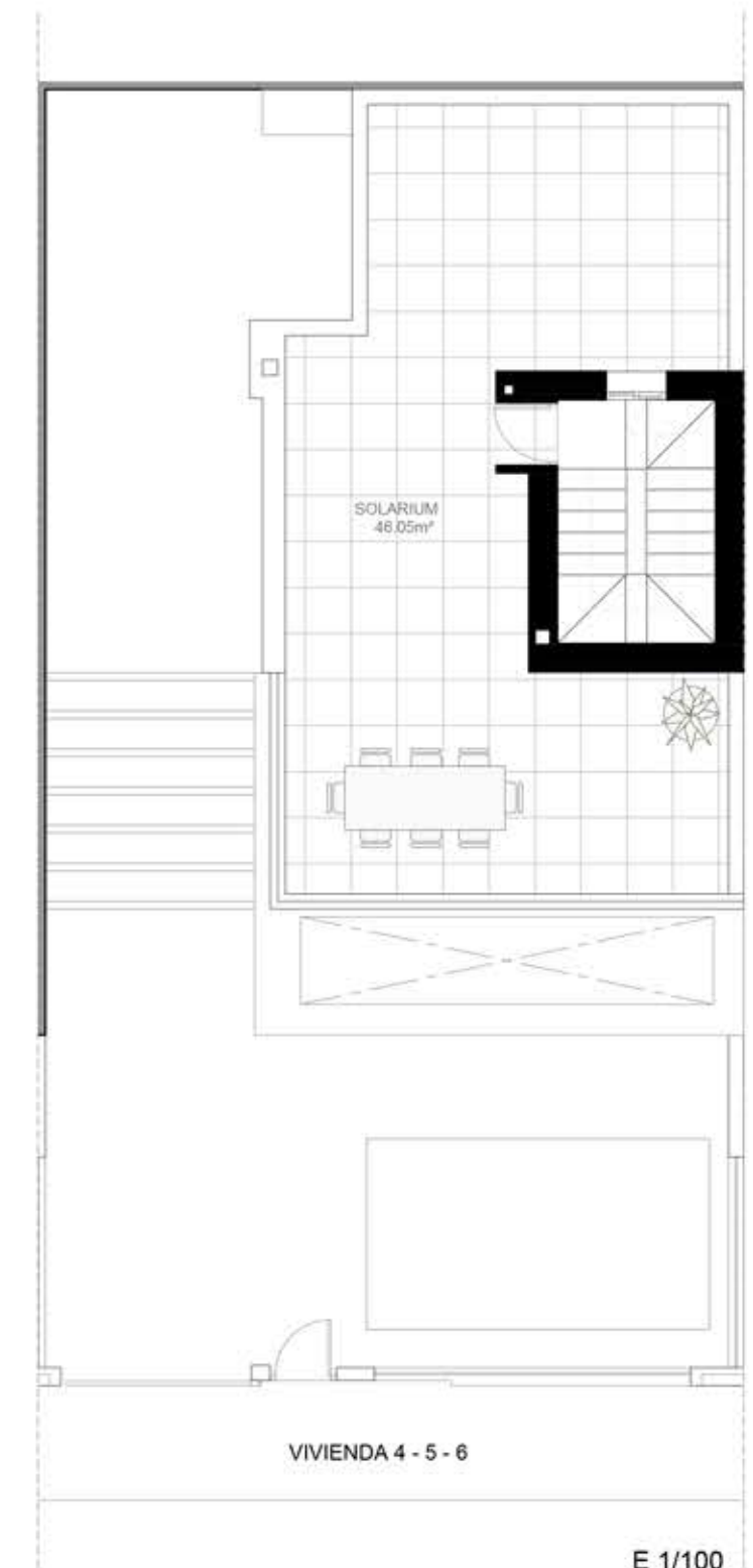
PLANTA SOLARIUM
