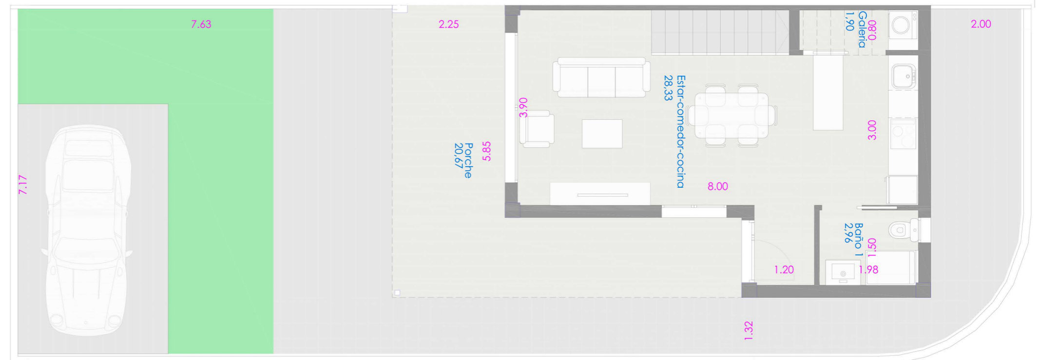
PLANTA BAJA
