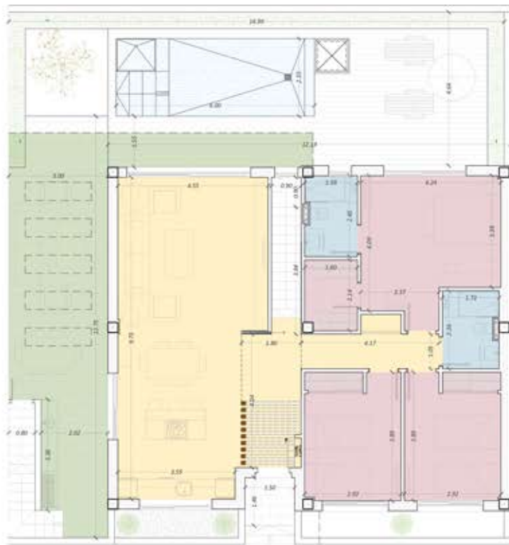
PLANTA BAJA
