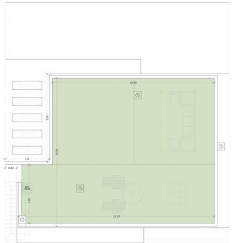
PLANTA CUBIERTA-SOLARIUM
