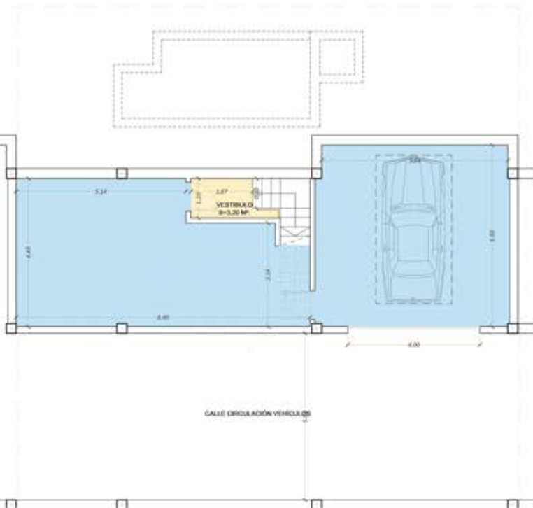
PLANTA SOTANO
