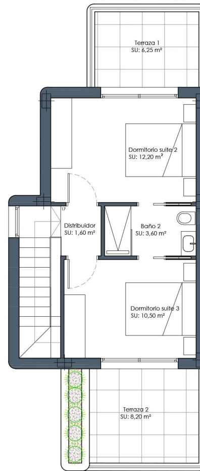
PLANTA PRIMERA
