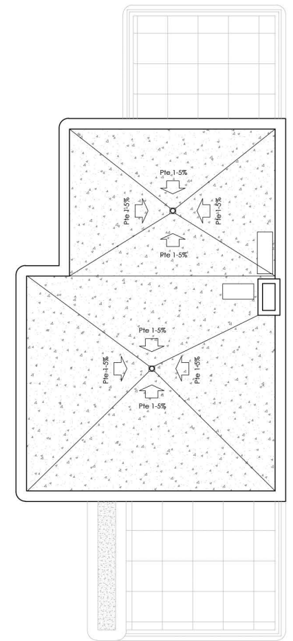
PLANTA CUBIERTA
