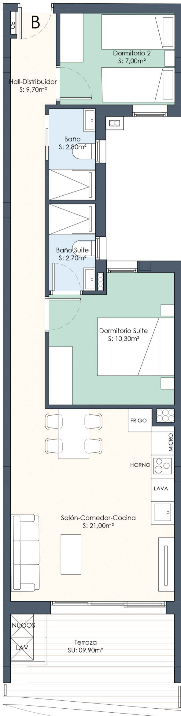
Planta Vivienda
